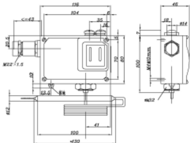
02 图 BL-W541-A(防爆)
