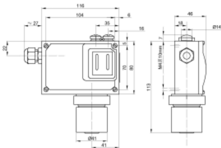
03 图 BL-W541-B(防爆)
