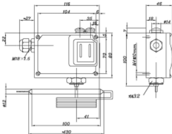
01 图 BL-W541-A
